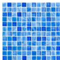
JSW-2312 Sheet Size : 300×300mm Chip Size : 23×23×6mm
